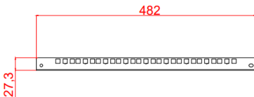
Вид спереди
