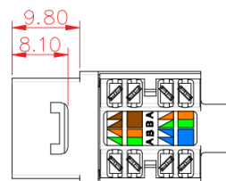
Вид снизу/сверху
