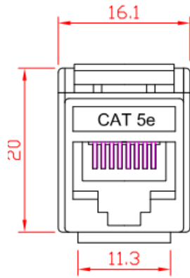
Вид спереди
