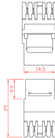
Вид снизу/сверху
