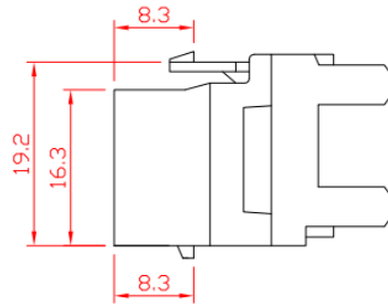
Вид сбоку
