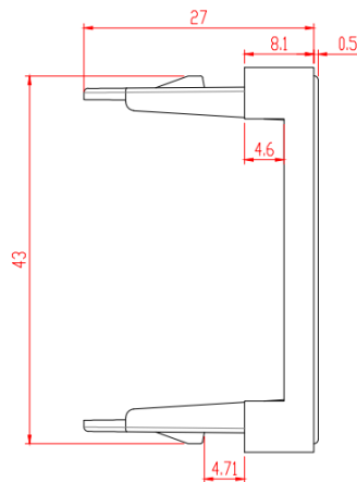
Вид сбоку
