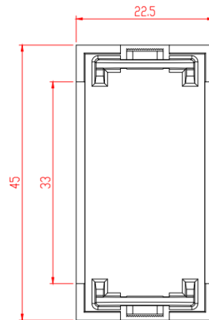
Вид сзади
